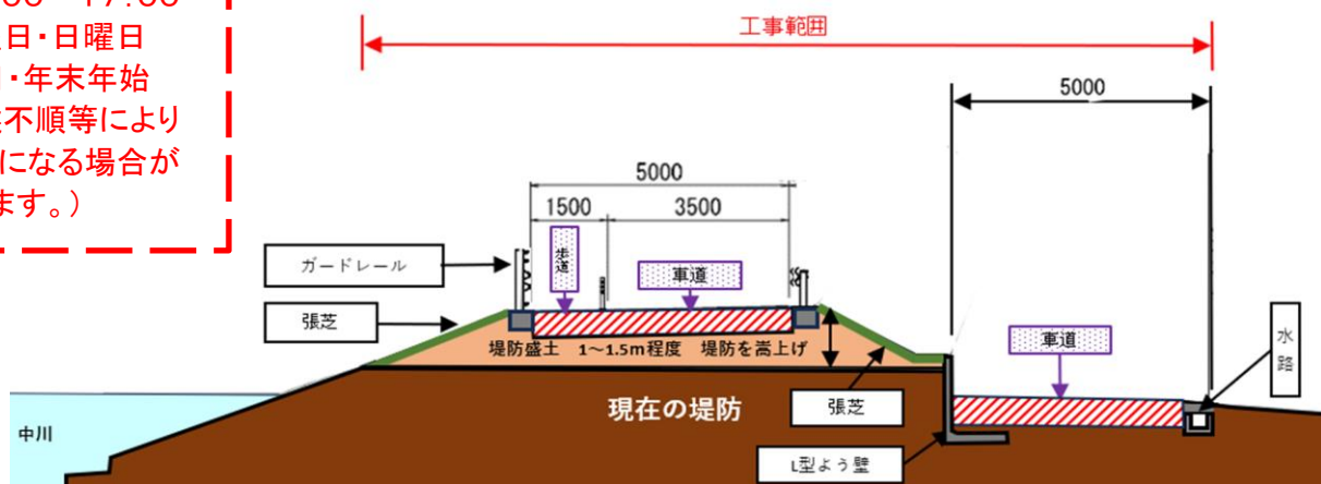
施工断面図（イメージ）
